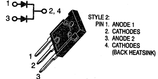
Case 340F (TO-247)
