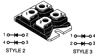
SOT-227B
